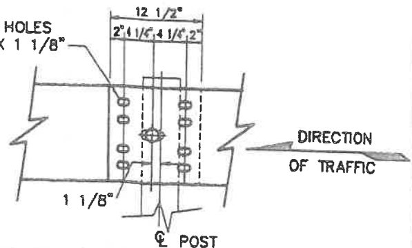
BEAM ELEMENT SPLICE N.T.S.
