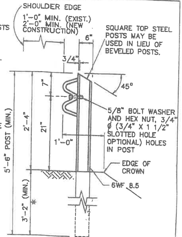
STEEL LINE POST N.T.S.
