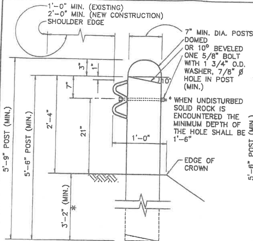
WOOD LINE POST N.T.S.
